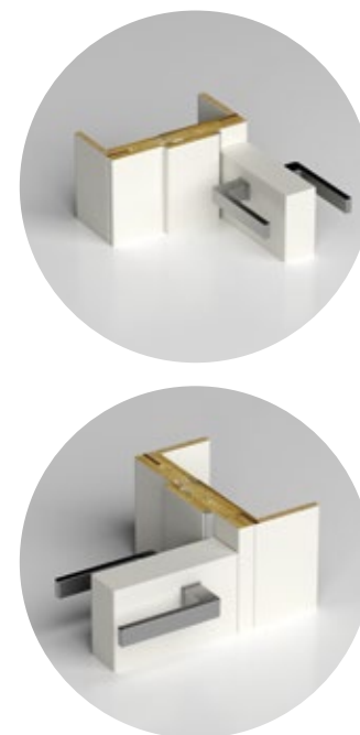
Telaio TX Per muri superiori a 15 cm for walls above 15 cm
