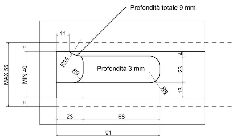
Dettaglio F
